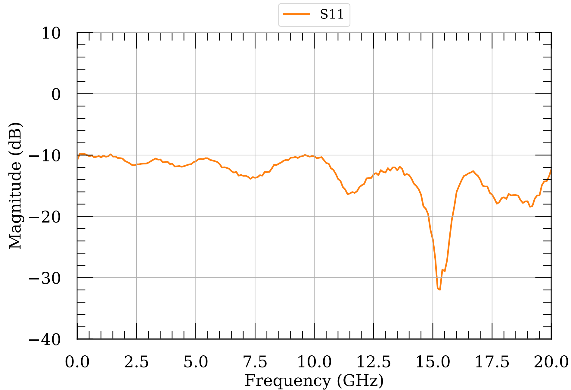
LNA S-params module086
